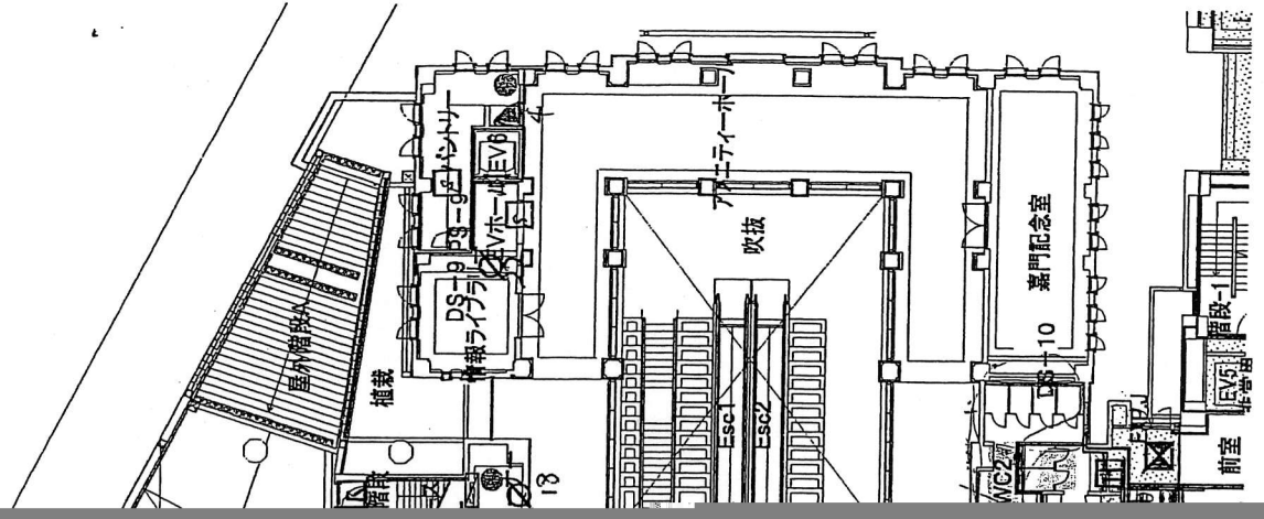
避難経路図 北棟2F
